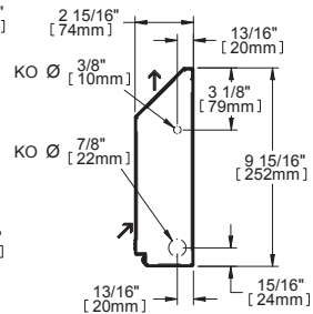
CÔTÉ | SIDE
