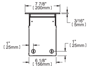
CÔTÉ | SIDE
