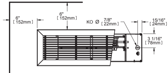
DESSUS | TOP
