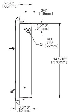
CÔTÉ | SIDE
