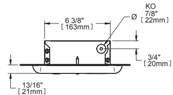
DESSUS | TOP
