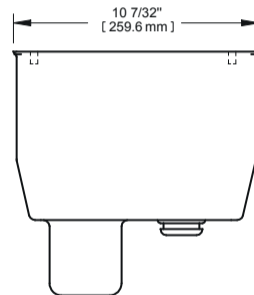
DESSUS | TOP
