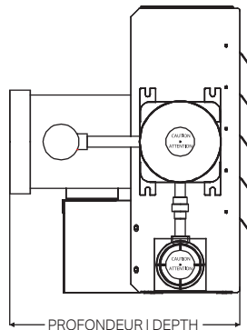
CÔTÉ | SIDE
