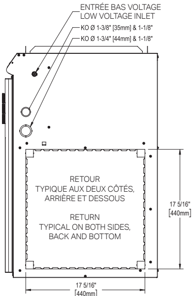
CÔTÉ | SIDE
