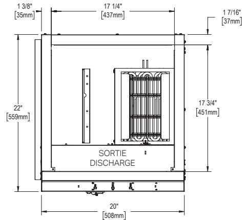
DESSUS | TOP
