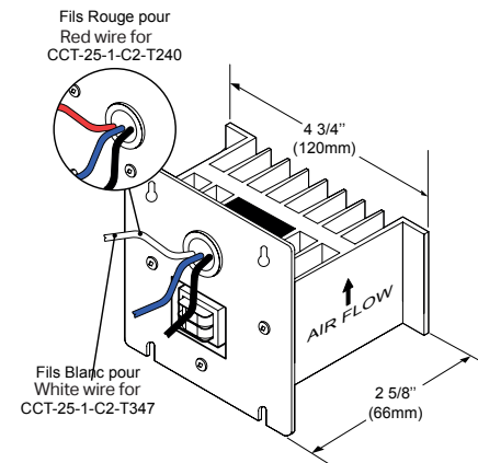
VUE ISOMÉTRIQUE / ISOMETRIC VIEW | CCT-25-1-C2-(T347), (T240)
