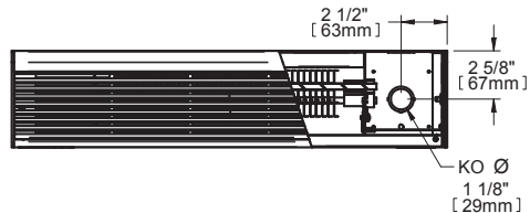
DESSUS | TOP
